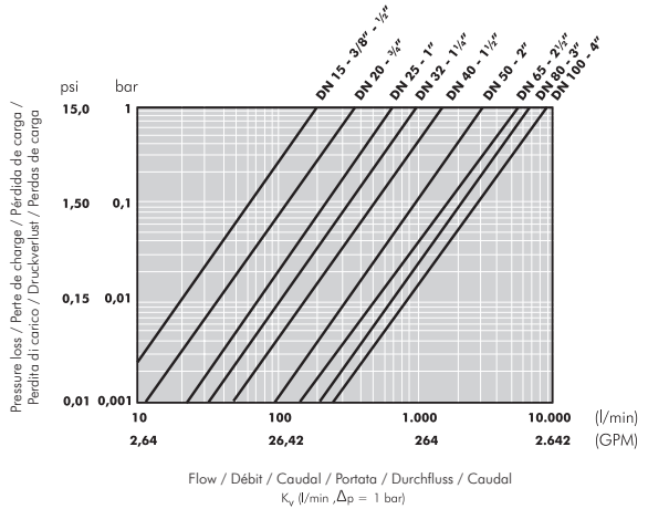
Diagramme de perte de charge (G 3.3)
